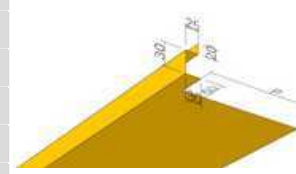
Détail linteau de fenêtre
