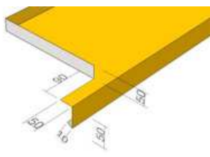
Détail appui de fenêtre
